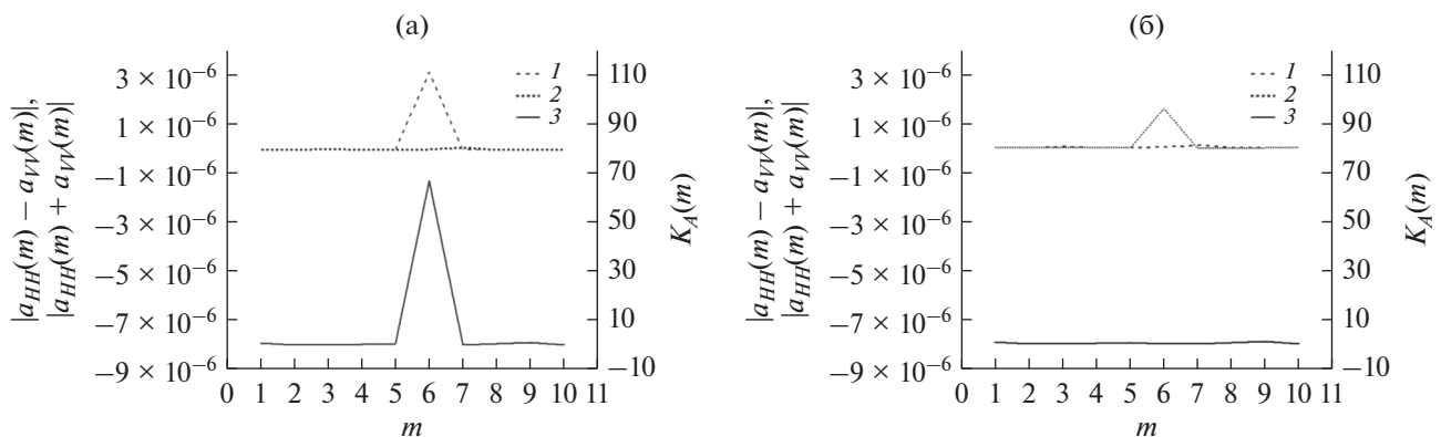
Рис. 4. Параметры и контраст Паули отражателя в терминах комплексных амплитуд: а – перпендикулярно плоскости ХОZ; б – повернут на 45^\circ вокруг оси x; |a_{HH}(m) - a_{VV}(m)| (кривая 1), |a_{HH}(m) + a_{VV}(m)| (кривая 2), K_A(m) (кривая 3).
