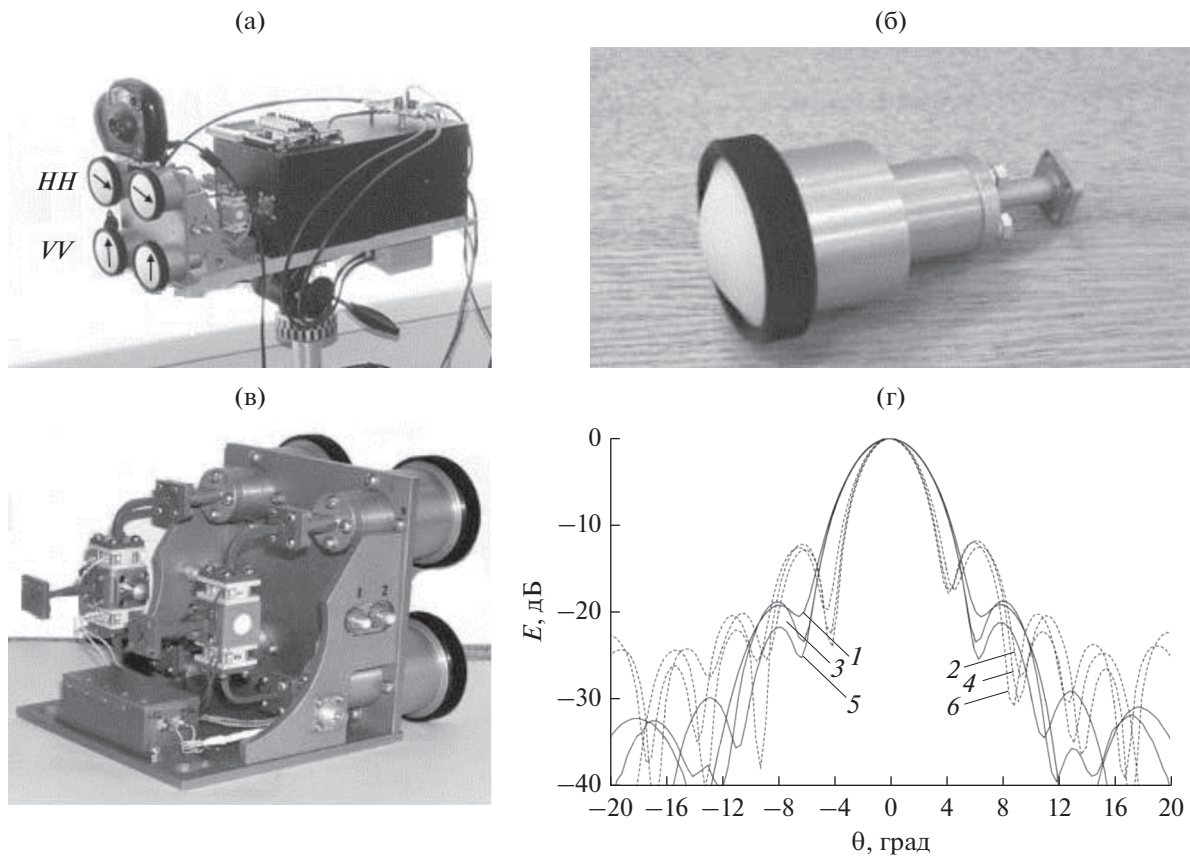
Рис. 7. Макет РЛСБД: а – приемоизлучающий тракт; б – рупорная антенна; в – высокочастотная часть макета; г – диаграммы направленности антенн: H плоскость (кривые 1, 3, 5); E – плоскость (кривые 2, 4, 6) на частотах 92, 93, 94 ГГц соответственно.
