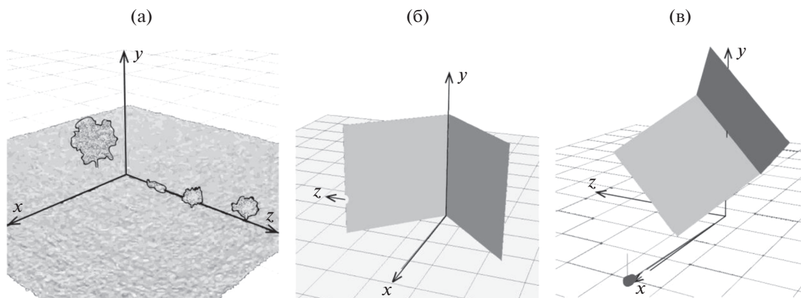
Рис. 1. Радиолокационные сцены: а – подстилающая поверхность, б, в – двугранный уголкового отражателя в двух положениях.
